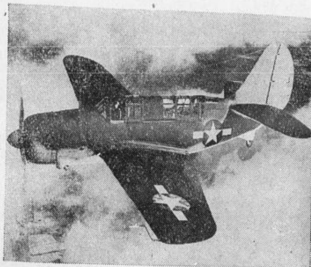
BOMBARDEIRO EM PICADA — A fotografia mostra um "HELLDIVER", último tipo de bombardeiro em picada das forças armadas norte-americanas. Este aparelho pode transportar maior carga de explosivos a grandes distâncias, manobrando tanto de terra como de bordo de porta-aviões. Por ocasião de seu "batismo de fogo" estes poderosos bombardeiros afundaram três navios de guerra japoneses na baía de Rabaul.
